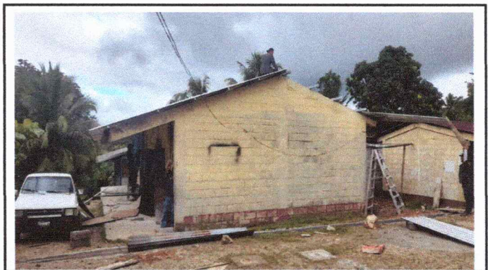
Foto 4: Se observa la colocación de cubierta de lámina troquelada en calibre "26
